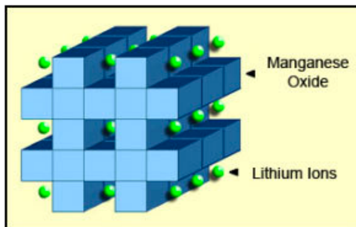
Figuur 4: Li-mangaanstructuur.
