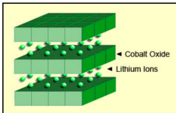
Figuur 1: Li-kobaltstructuur.
